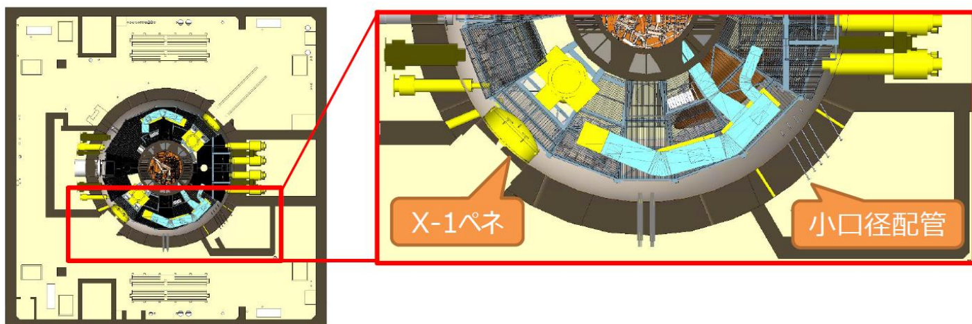
図1 PCV 内部調査の対象箇所
