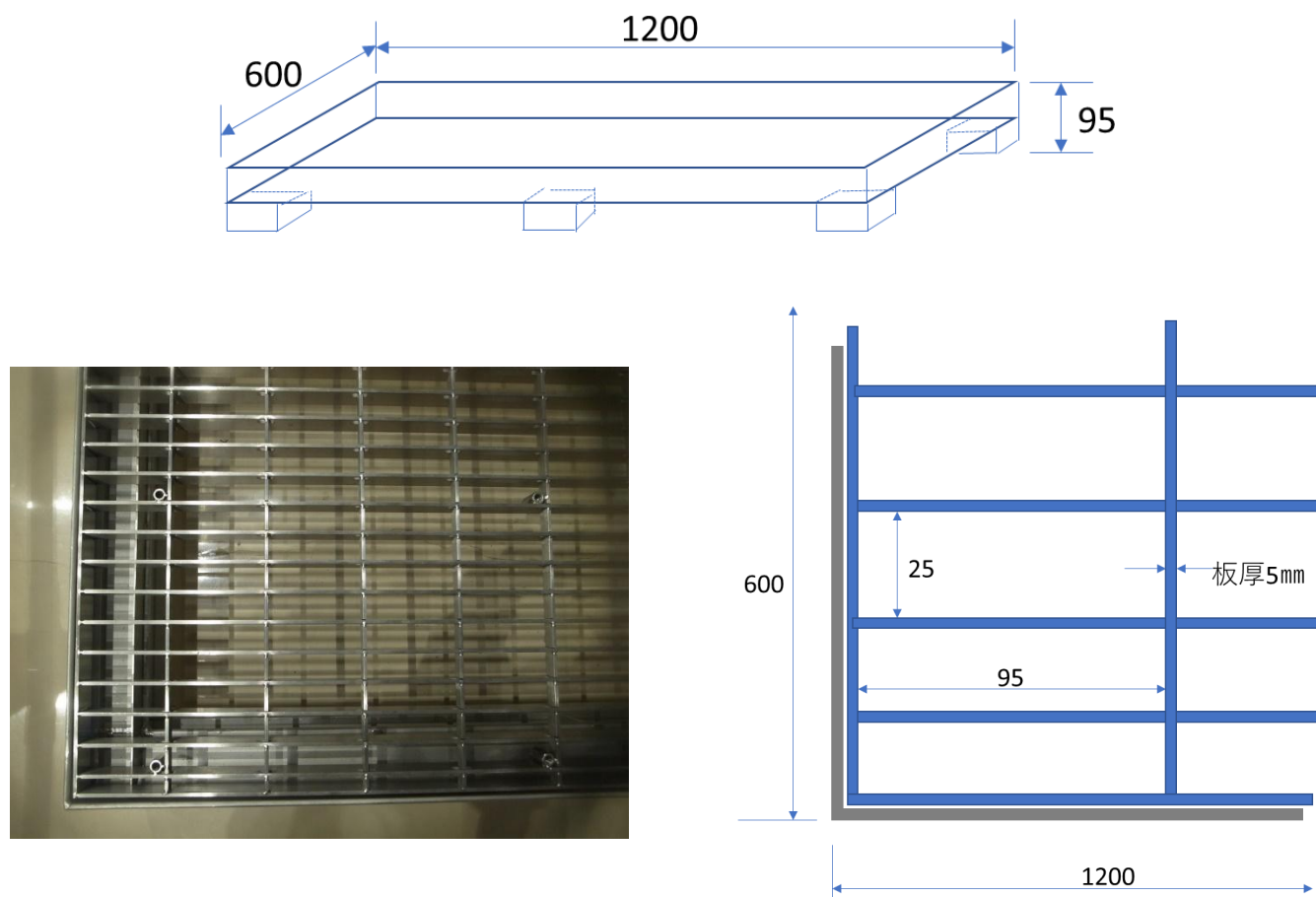
図4 グレーチング
